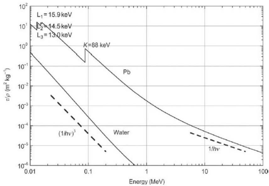
Figura 3: Sezione d'urto per acqua e piombo.
