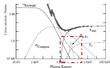
Sezione d'urto per reazioni fotonucleari: Esempio di risonanza gigante in Piombo, picco a 13,6 MeV
